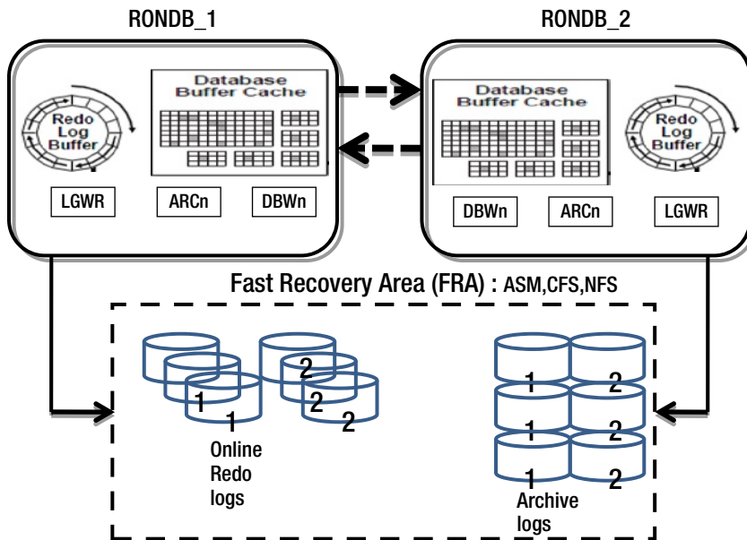
Figure 8-3. FRA settings
